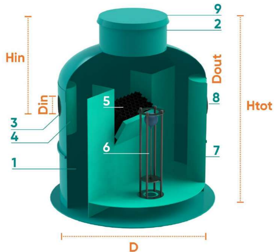
Fig. 1 Separador de hidrocarburos Vodaland OilBase 100 A – Cámara de lodos; B – Cámara coalescente
